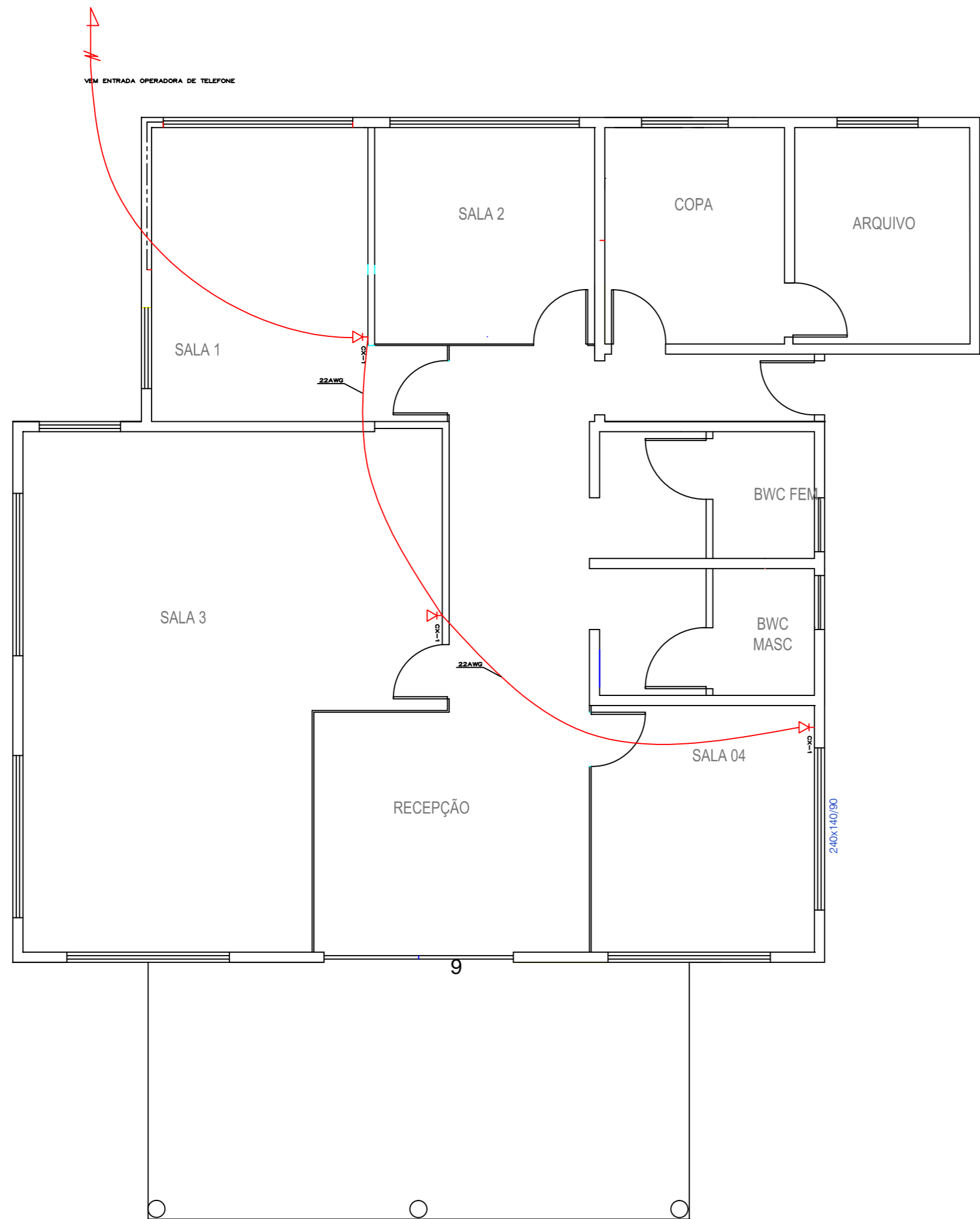
PLANTA TELEFONICO ESCALA 1:75
